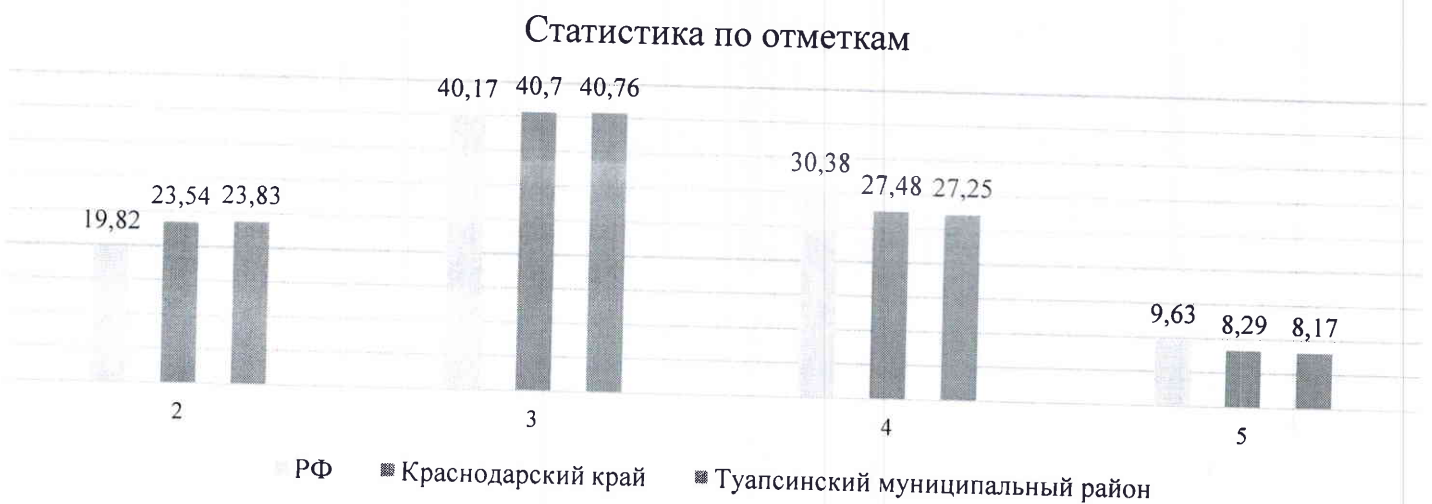
Рис. 1. Статистика по отметкам
