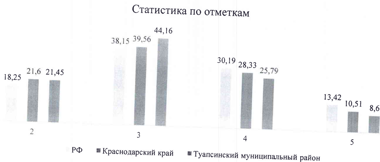
Рис. 1. Статистика по отметкам
