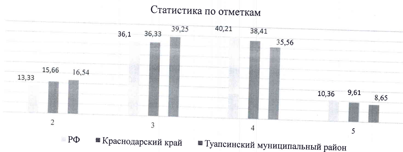
Рис. 1. Статистика по отметкам
