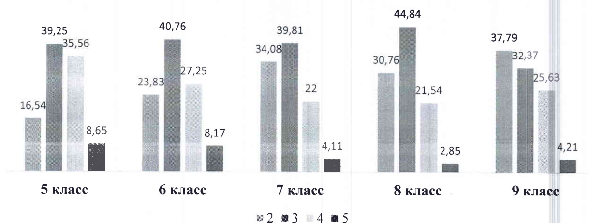
Рис.1. Динамика изменения отметок по классам
