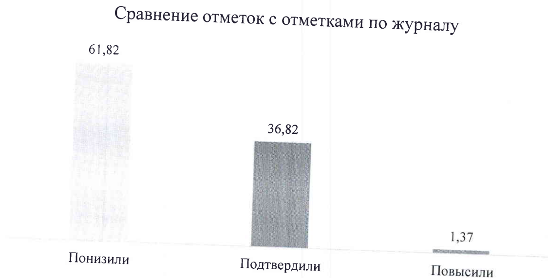
Рис. 2. Соответствие отметок за выполненную работу и отметок по журналу
