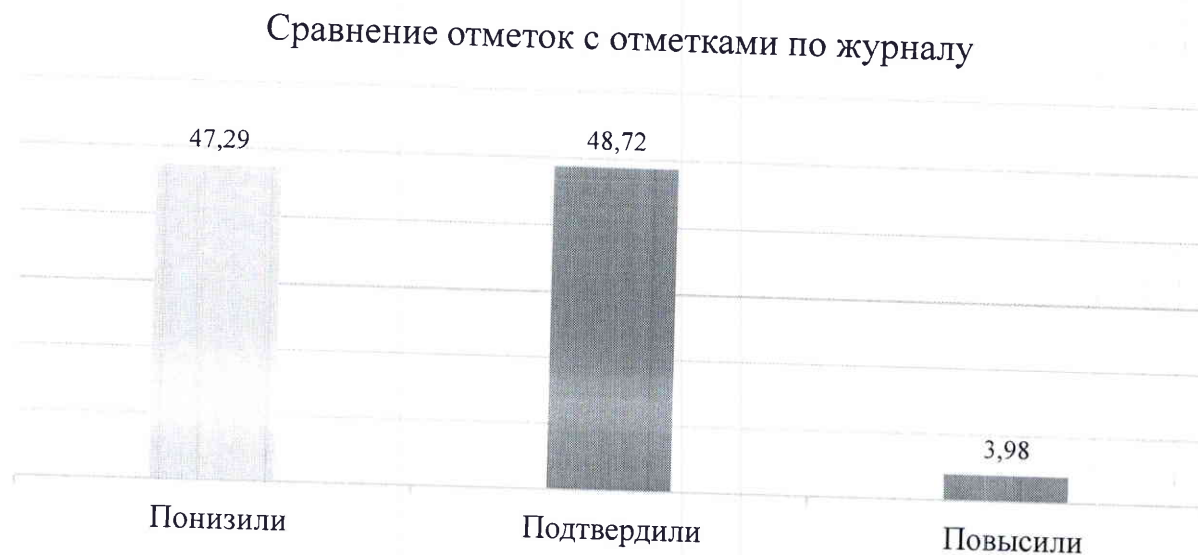
Рис. 2. Соответствие отметок за выполненную работу и отметок по журналу
