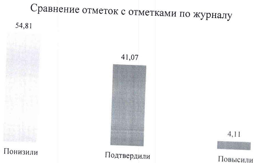
Рис. 2. Соответствие отметок за выполненную работу и отметок по журналу
